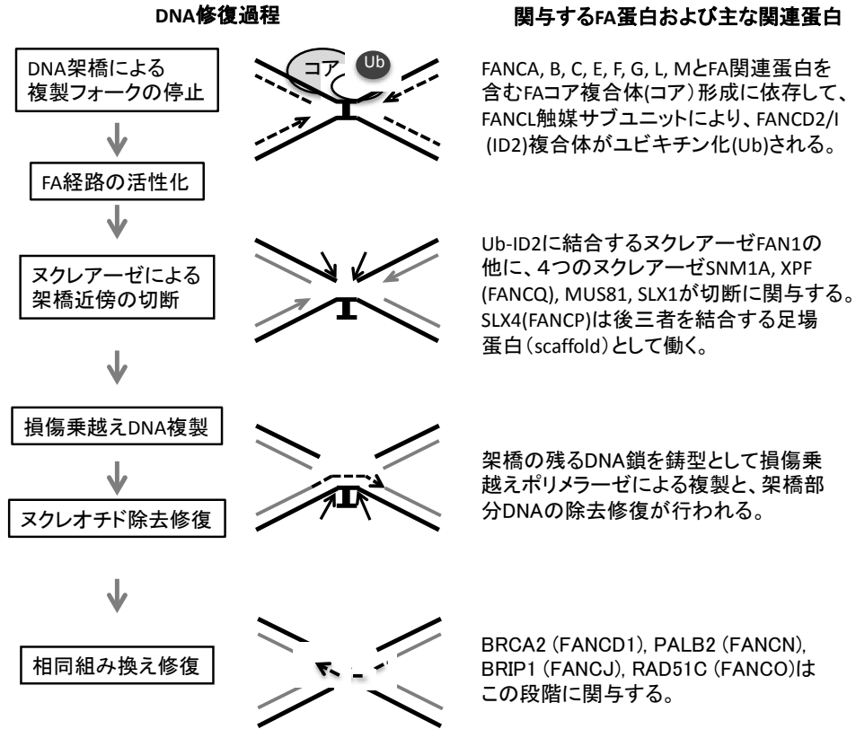
図2 FA経路の活性化とDNA架橋の修復モデル
